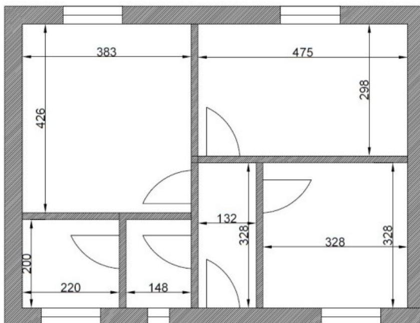
Slika 3 - Tlocrt stana
